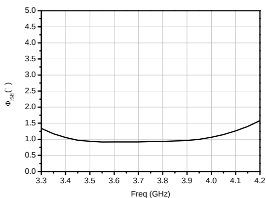
移相幅度波动
