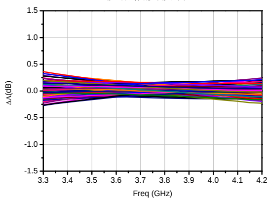
移相幅度波动
