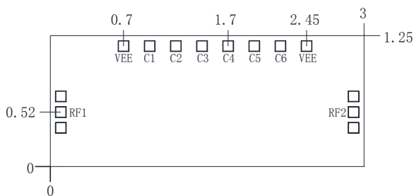
外形和端口尺寸 (mm)
