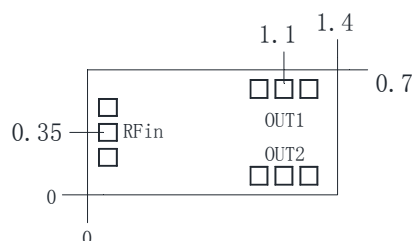
外形和端口尺寸 (mm)
