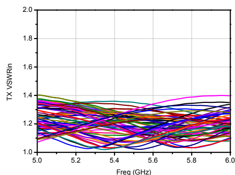
输出驻波
