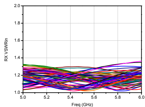
输入驻波
