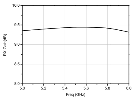
接收增益
