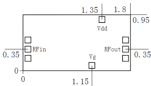
推荐装配图
