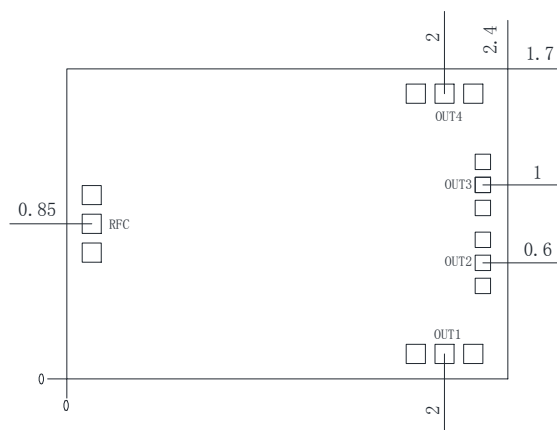
外形和端口尺寸 (mm)
