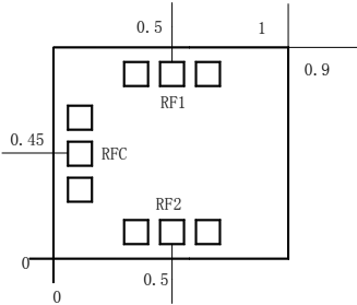
外形和端口尺寸 (mm)
