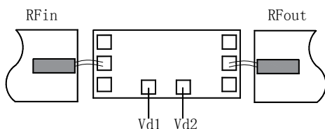
推荐装配图
