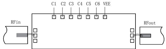
推荐装配图
