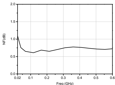
噪声系数
