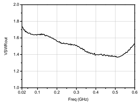
输出驻波
