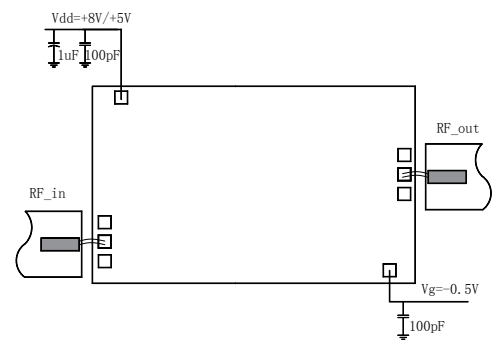
芯片装配示意图
