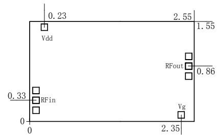
芯片装配示意图
